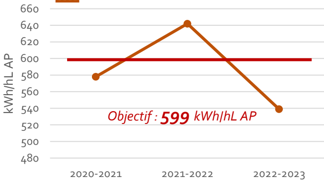
Consommation de gaz
