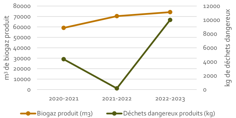
Suivi du biogaz produit par méthanisation et quantité de déchets dangereux traités
